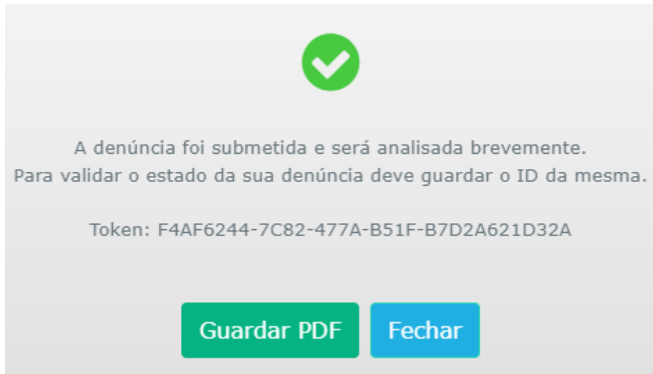
Figura 2 – Token
