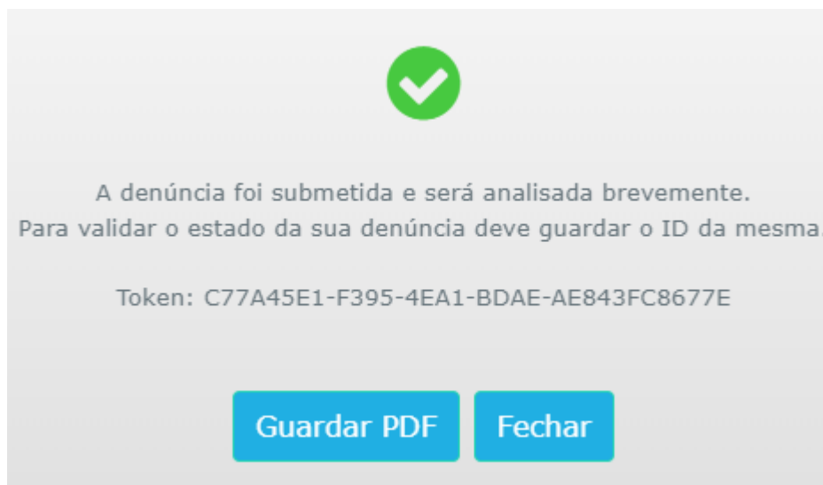
Figura 5 – Token
